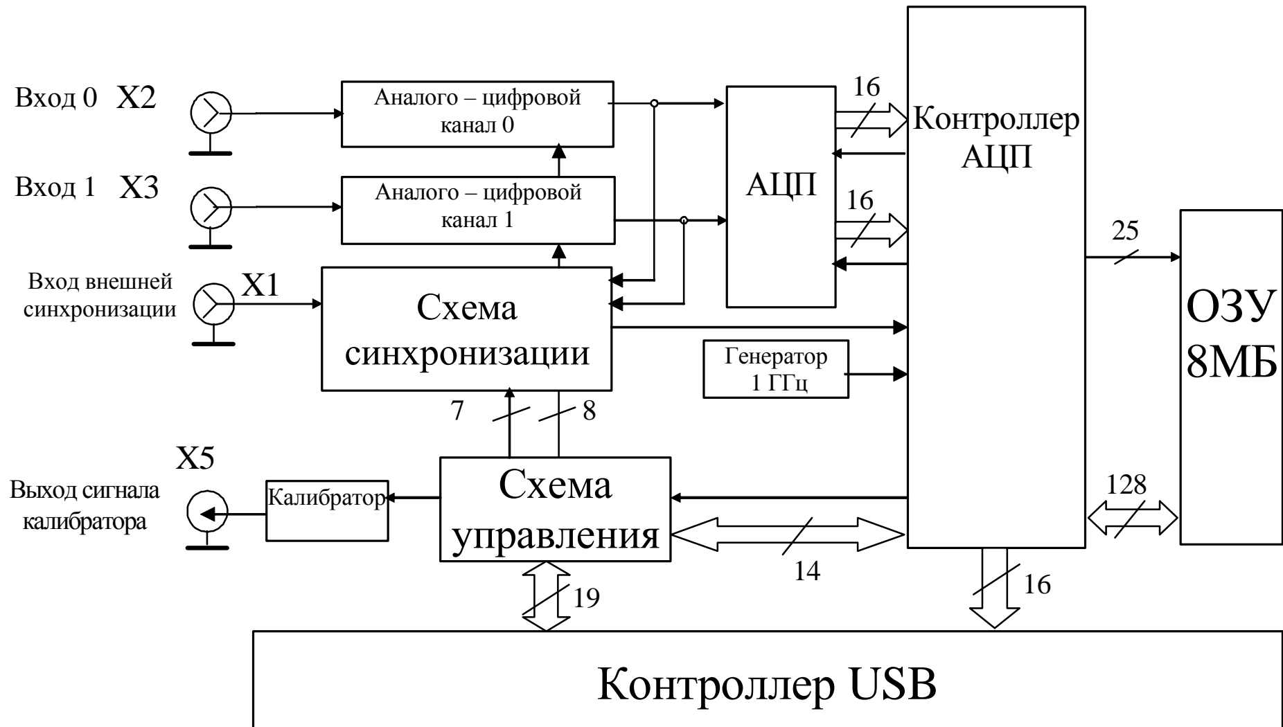
Рис. 5.1 Функциональная схема ОЦЗС-02(1000USB)
